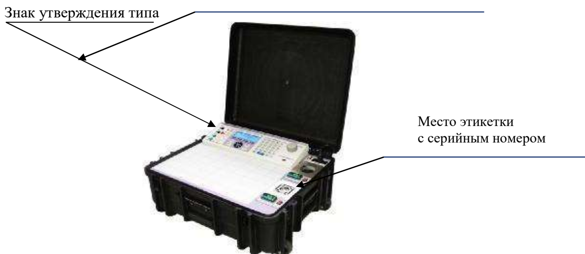
Рисунок 2 – Калибраторы многофункциональные 3041TR, 3050TR, место нанесения знака утверждения типа и серийного номера
