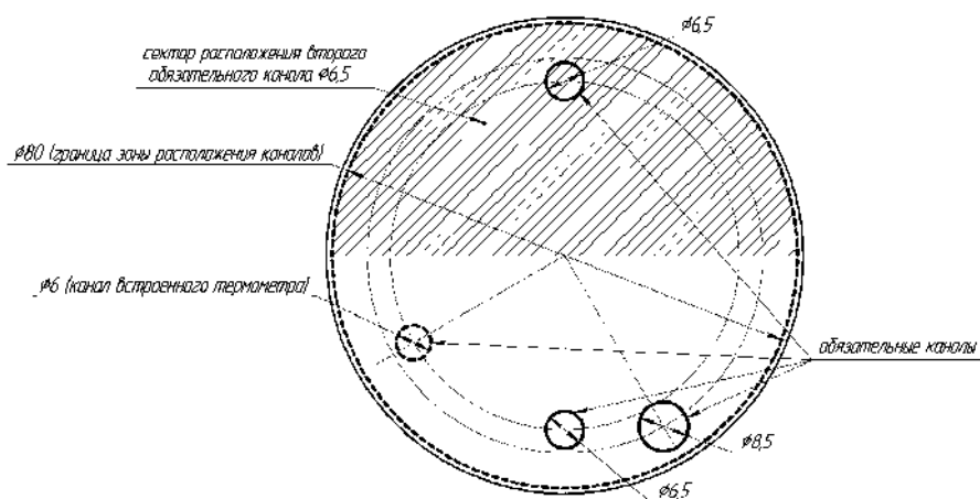
Рисунок А.2 — Эскиз термостатирующего блока ЭЛЕМЕР-КТ-650К/М1 для расположения нестандартного набора каналов (НТБ)
