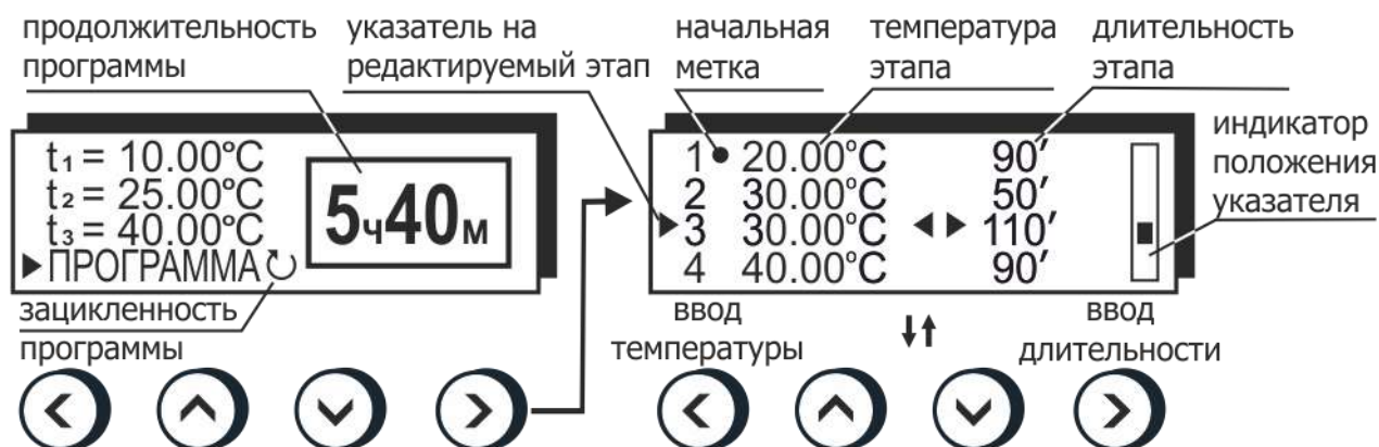
Рисунок 20 — Редактирование программы
