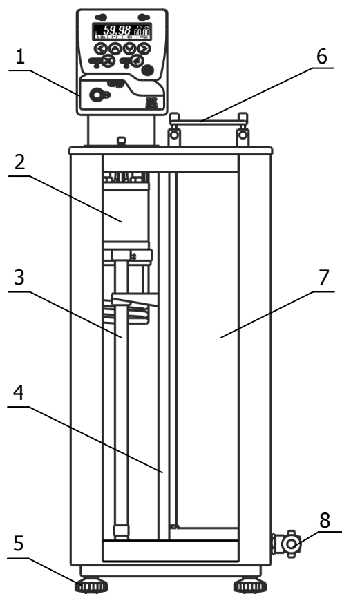
Рисунок 1 — Устройство термостата
