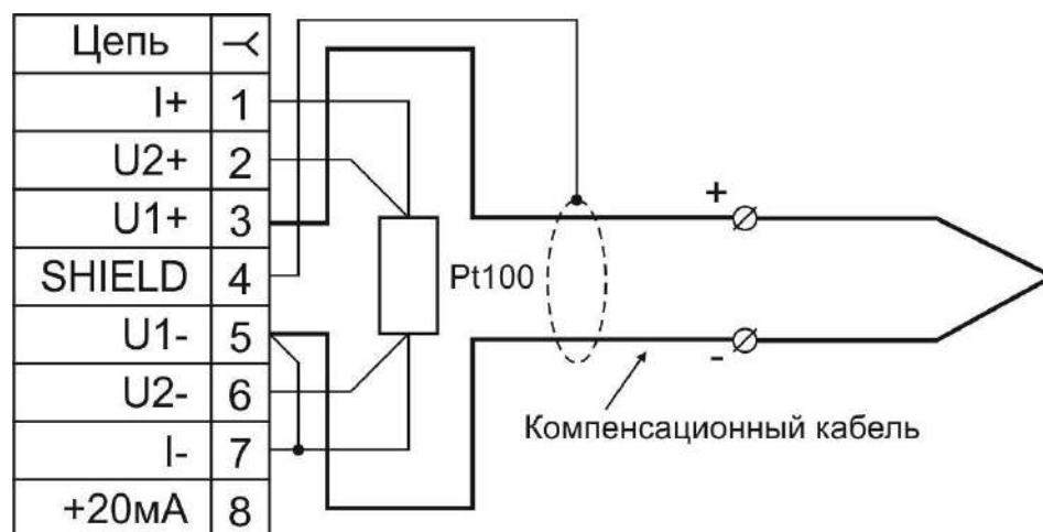
Рисунок Б.3 – Соединительный кабель № 03 для подключения термопреобразователей термоэлектрических с НСХ ТХА(К) и ТХК(Л). Компенсационный кабель с компенсатором холодного спая, установленным в разъеме
