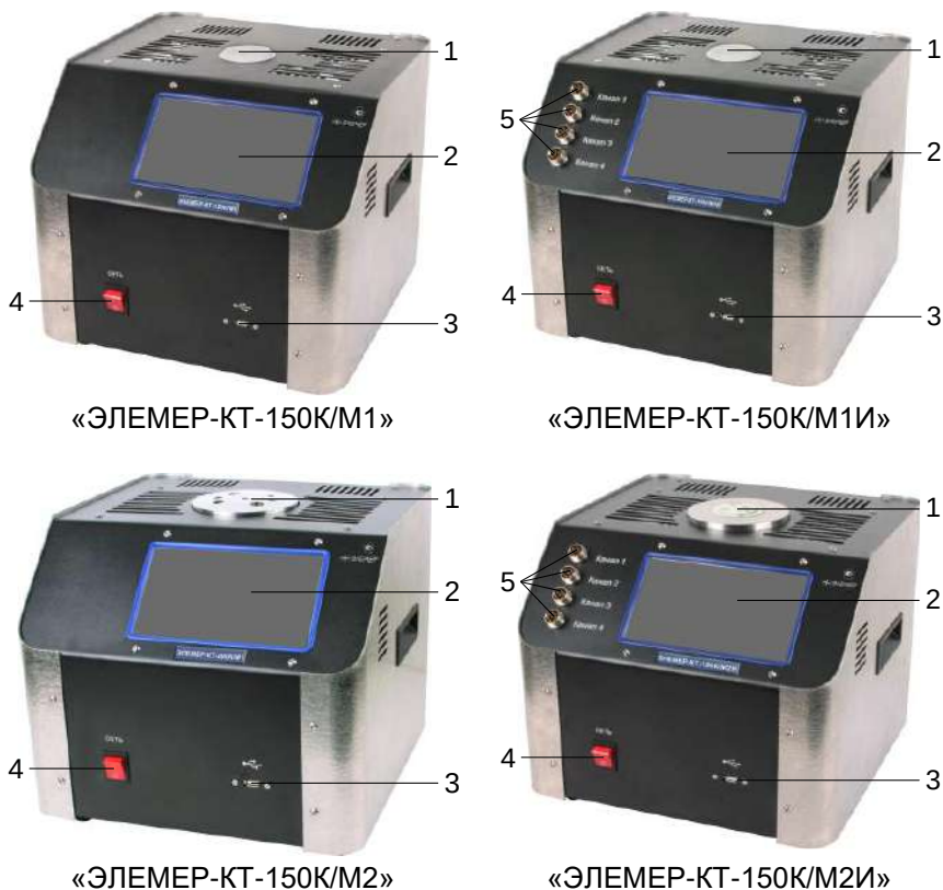
Рисунок 5.1 - Общий вид калибраторов
