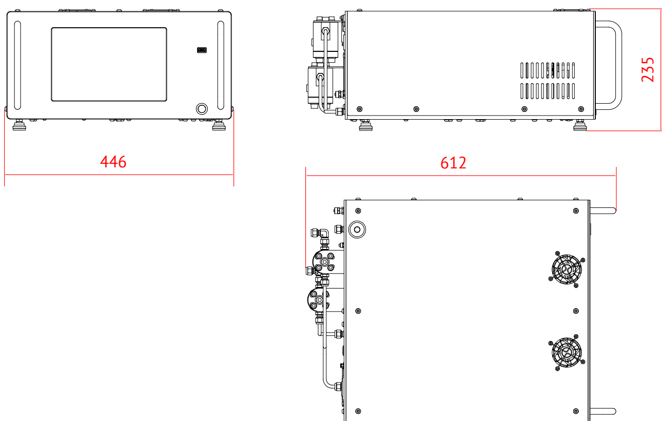
Рис. 1. Блок управления.
