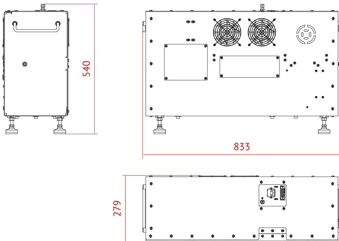
Рис. 2. Силовой блок.
