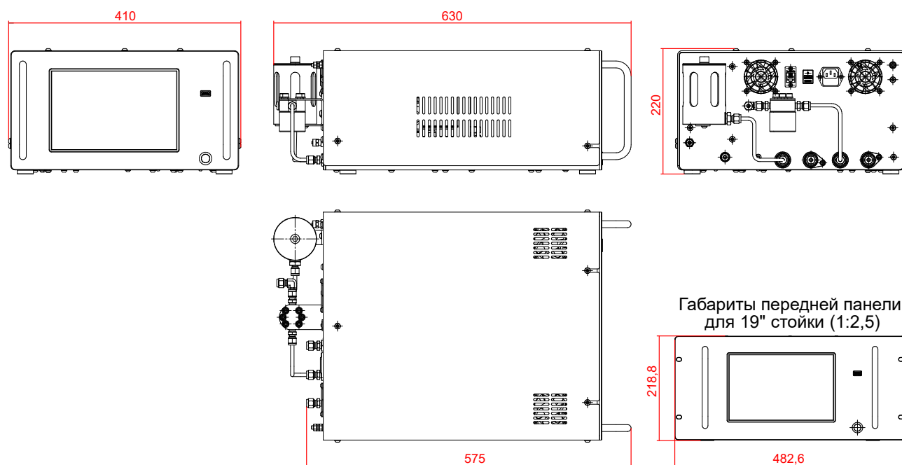
Рис. 1. Автоматический калибратор-контроллер давления АПК.
